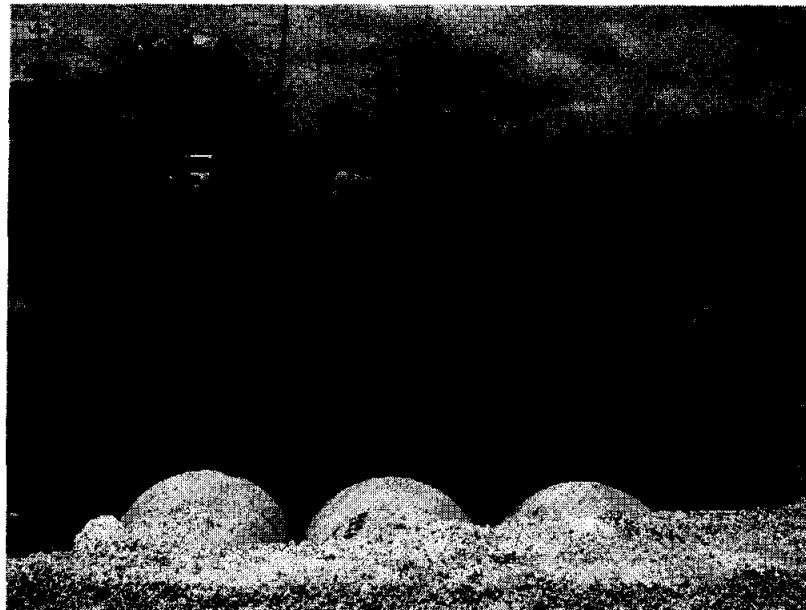
Fotos 1-2. Instalación tubería de drenaje
